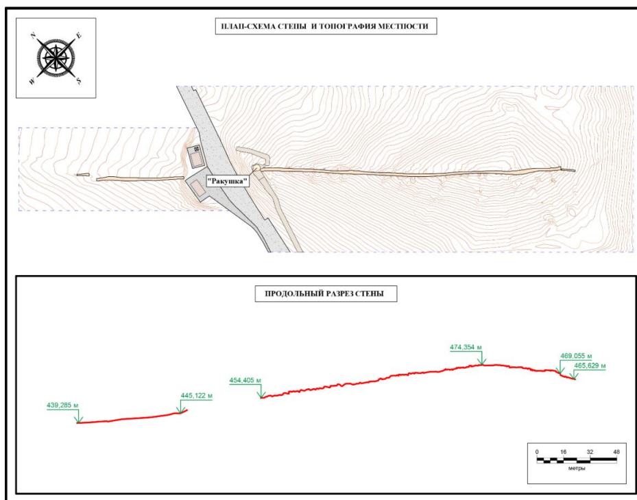
Рисунок 3. Рис. 3. План-схема западной стены комплекса Таскамал и топография местности
