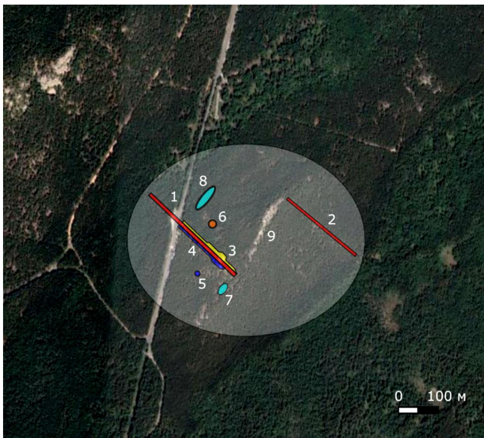
Рисунок 2. План-схема комплекса Таскамал: 1. Западная стена; 2. Восточная стена; 3. Терраса и пандусы; 4. Внешний участок; 5. Южная площадка; 6. Мастерская; 7-8. Горные выработки; 9. Природный скальный хребет.
