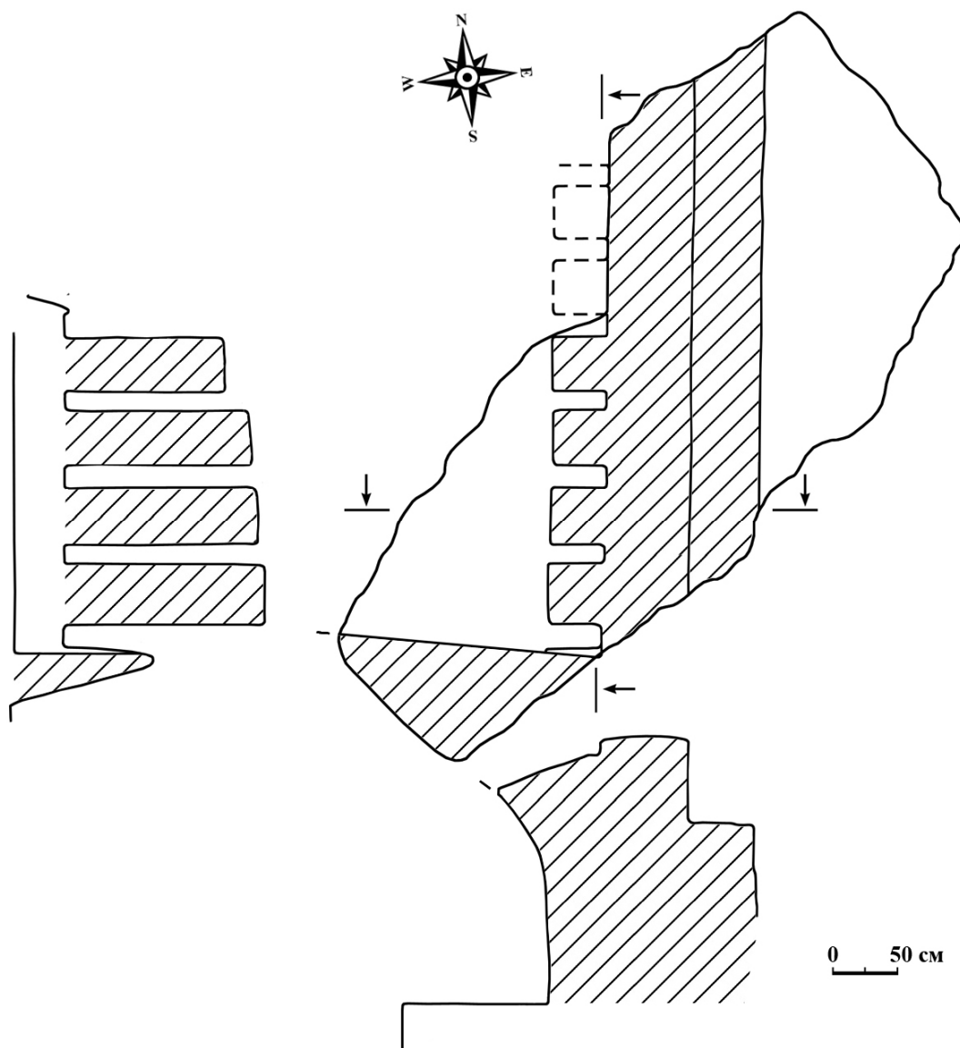
1-сурет. Сортобе кірпіш күйдіретін пеші. Жоспары
