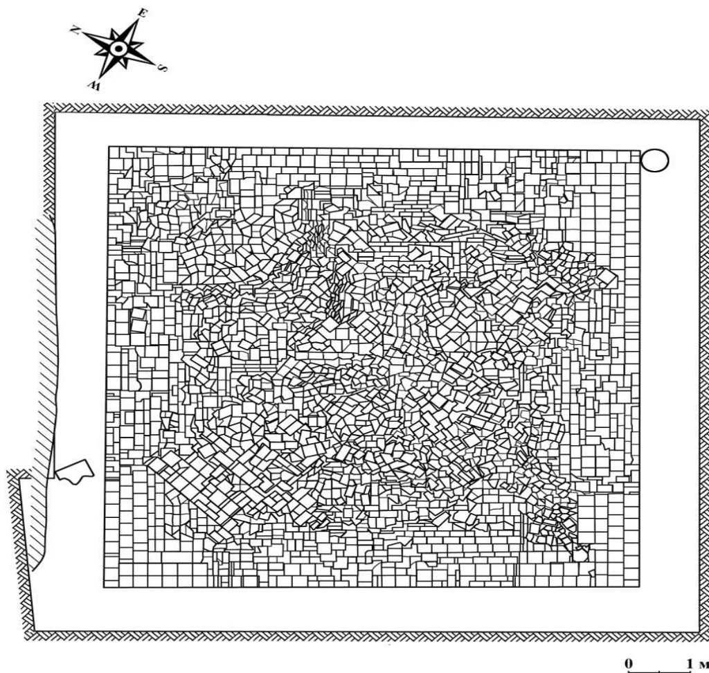
Ақтөбе қаласы. Мұнара іргетасы жоспары
