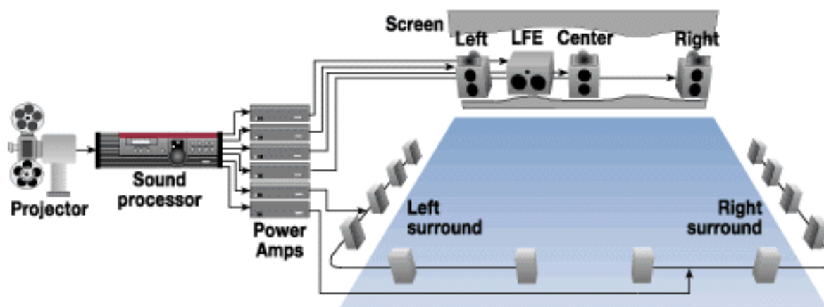
Рис.№1. Система DolbyDigital
