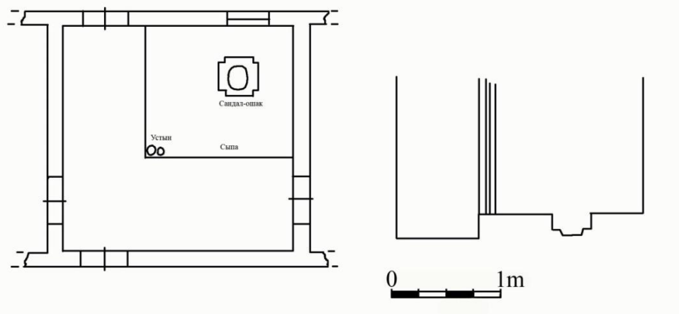
Сурет 6 – Сандал-ошақ орналасқан бөлменің сызбасы.
